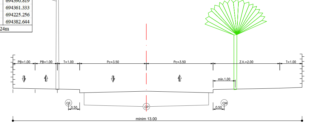
PROFIL TRANSVERSAL PROPUȘ E - E STR. INDUSTRIILOR
