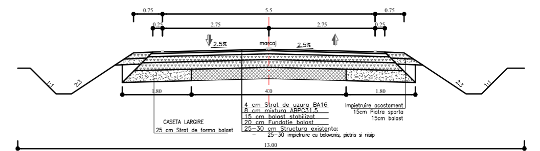
PROFIL TRANSVERSAL E - E CONFORM PROIECT TEHNIC DE EXECUȚIE IMPLEMENTAT STR. INDUSTRIILOR
