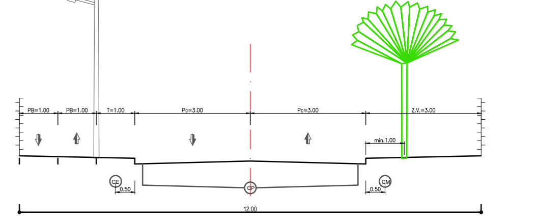
PROFIL TRANSVERSAL P - P DRUM PROPUȘ
